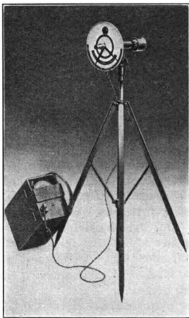
FIG. 4.—SCIMATCO PYROMETER.
