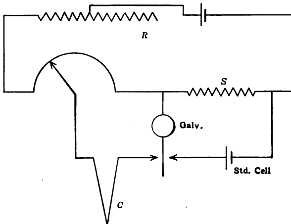
FIG. 2.—SIMPLE POTENTIOMETER CIRCUIT.
