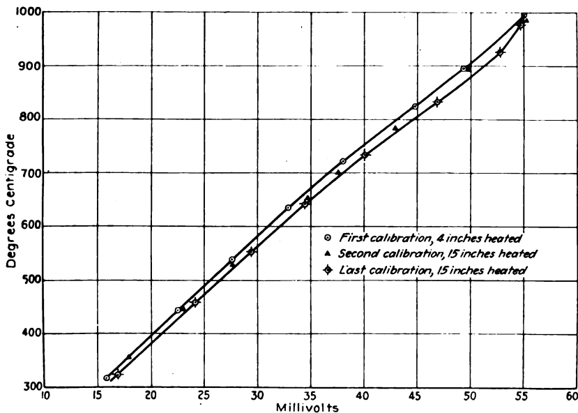
FIG. 3.—CALIBRATION OF COUPLE 20.
