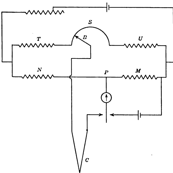
FIG. 3.—SPLIT-CIRCUIT POTENTIOMETER.
