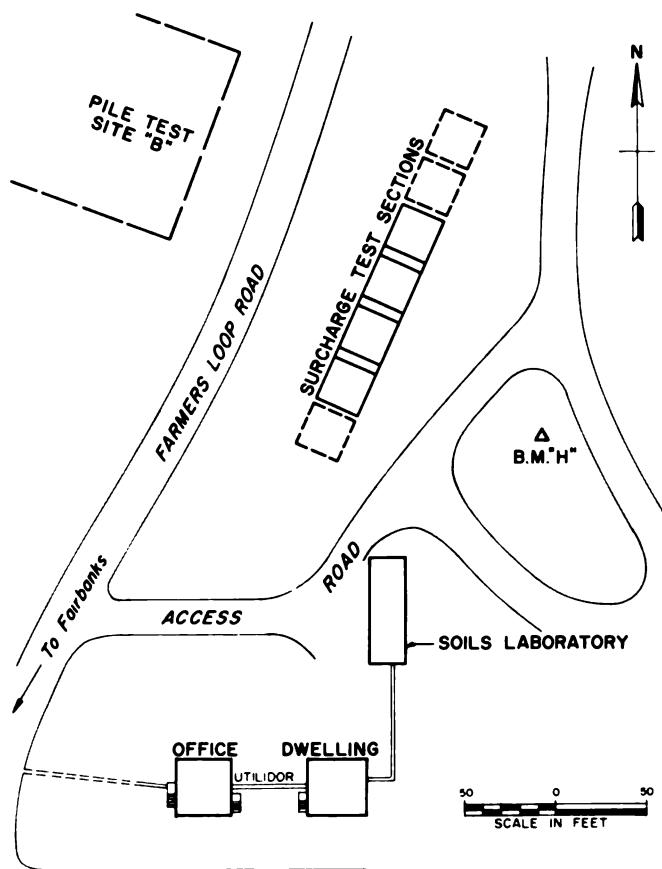
Fig. 1. Site layout
