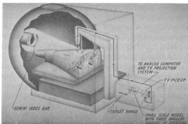
FIG. 4. Visual docking simulator.
